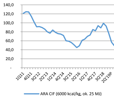
ARA [USD/t]
