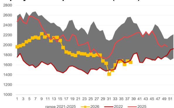
Zapasy diesla w portach ARA (k tons)
